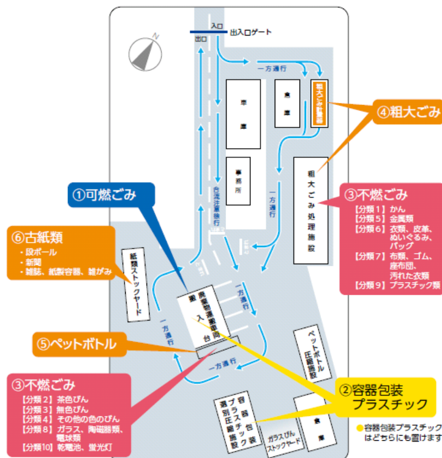
じん芥処理場内配置図
