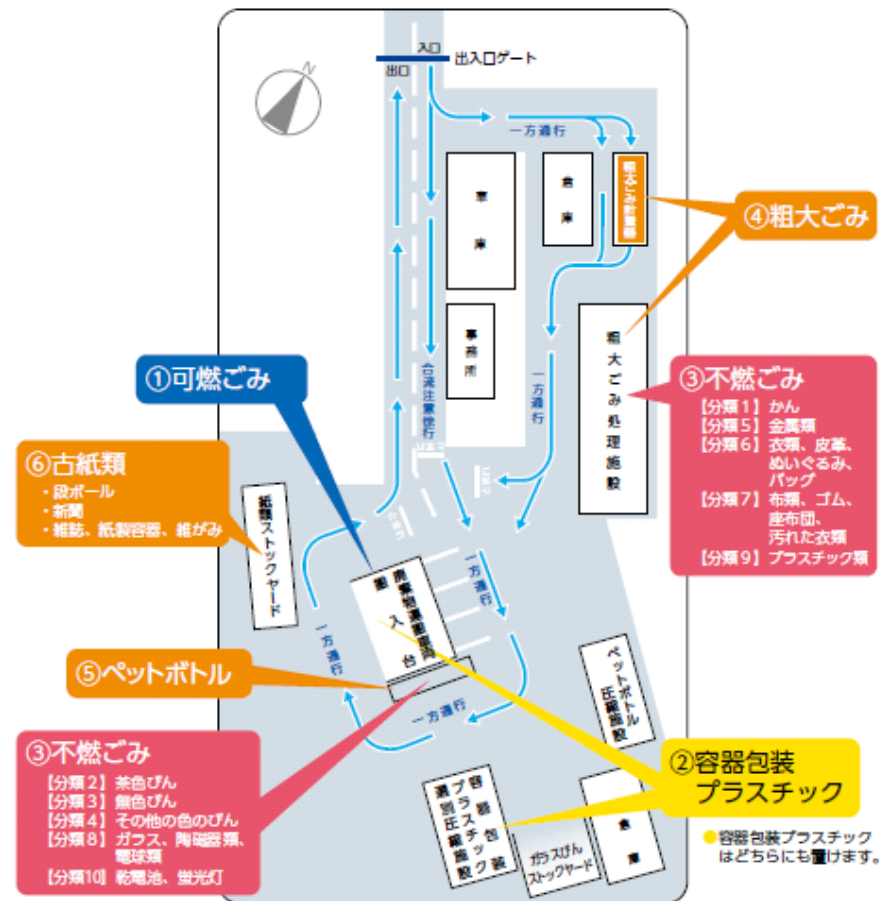
じん芥処理場内配置図
