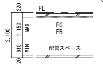
床下ピット位置を示す。断面図 S=1/100
