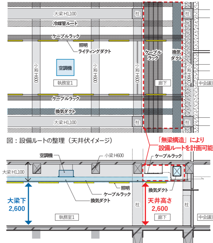
図：「無梁構造」を用いた廊下・執務室の断面イメージ
