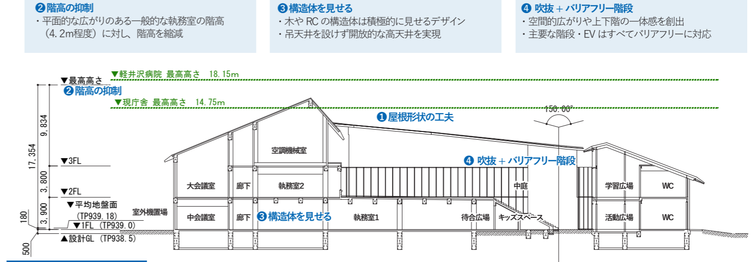
断面図2
