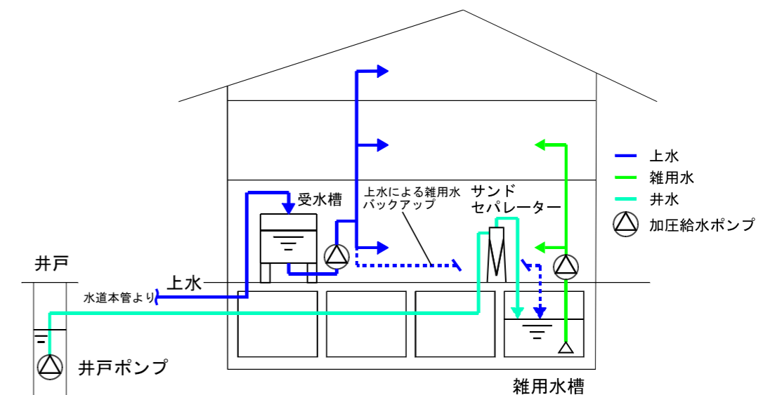
図：給水概略フロー図
