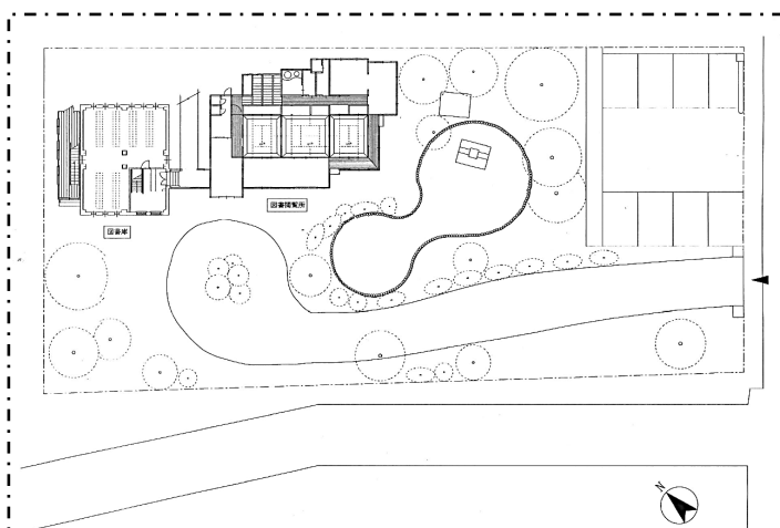
図 1-3 配置図(意見具申添付用)の作成例
