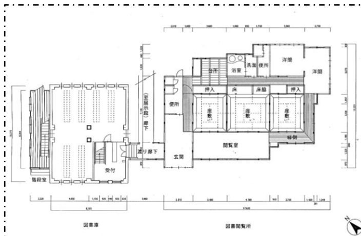
図 1-2 平面図の作成例
