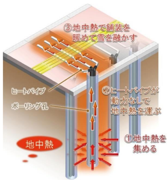
地中熱利用ヒートパイプイメージ図
