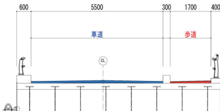
【断面図(標準部)】
