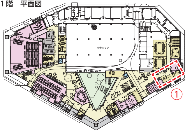
1階 平面図
